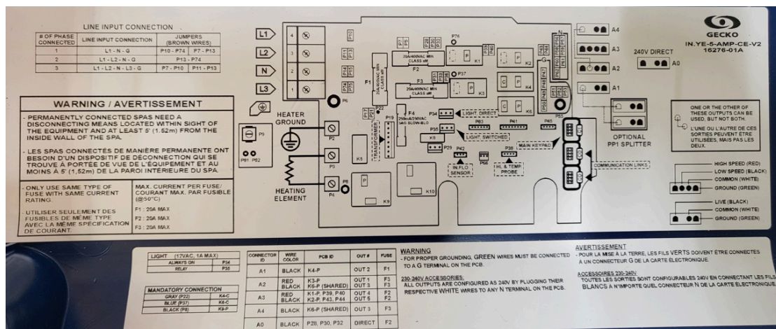
Schaltplan Anschlussbelegung & Jumper
