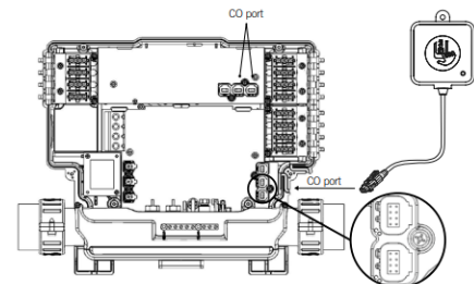
CO-Port an der Steuerbox
